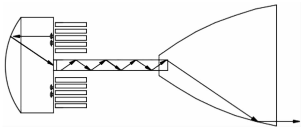
图 1 新型 LED 太阳模拟器光学结构示意图 Fig. 1 Optical structure diagram of a new type of LED solar simulator
