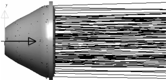
图 3 透镜光线追迹图 Fig. 3 Lens ray tracing 将光源设定为尺寸 1 mm×1 mm 的朗伯型光源,透镜材料设置为折射率 1.49 的聚甲基丙烯酸
