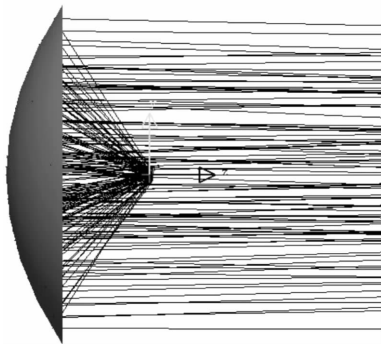
图5 抛物面镜聚光模拟
