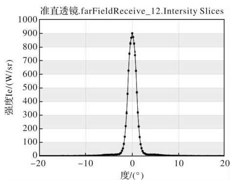
图4 准直后配光曲线
